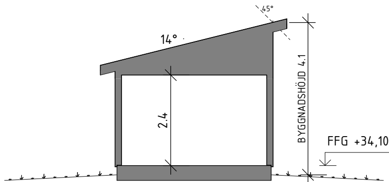
SEKTION A-A
